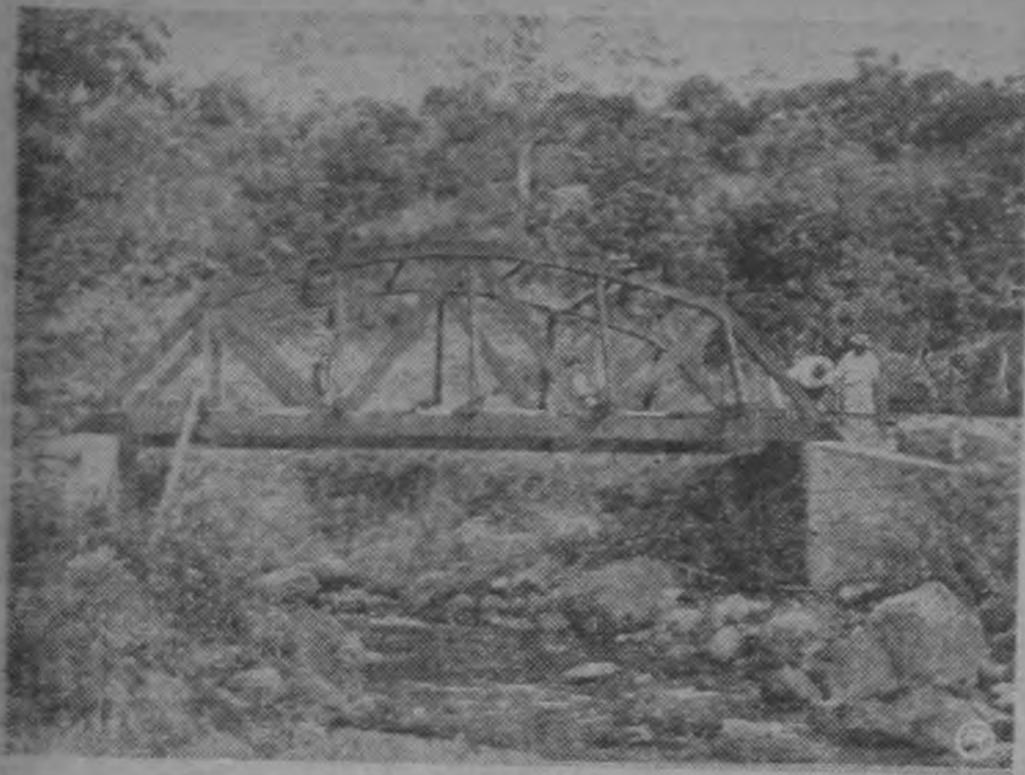
Una vista del puente sobre el río Palomo, en Palomo de Orosi, que será inaugurado en breve. Tiene 9 metros de largo, 3.10 m. de ancho. Ha sido construido en 9 semanas, con madera de Tirrá, prefabricado en el plantel de Obras Públicas de Cartago. Las platinas y varillas de hierro fueron hechas también en el Taller de Obras Públicas. Fue diseñado por el Ing. Luis Alberto Murillo. (FOTO COLO)
